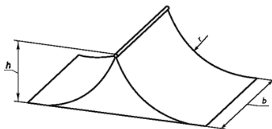
Рисунок 11 - Рампа с гребнем
