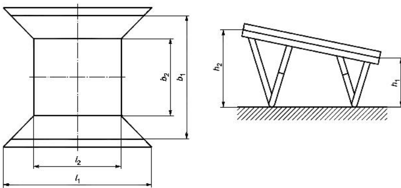
Рисунок 3 - Размеры батутов класса 3
