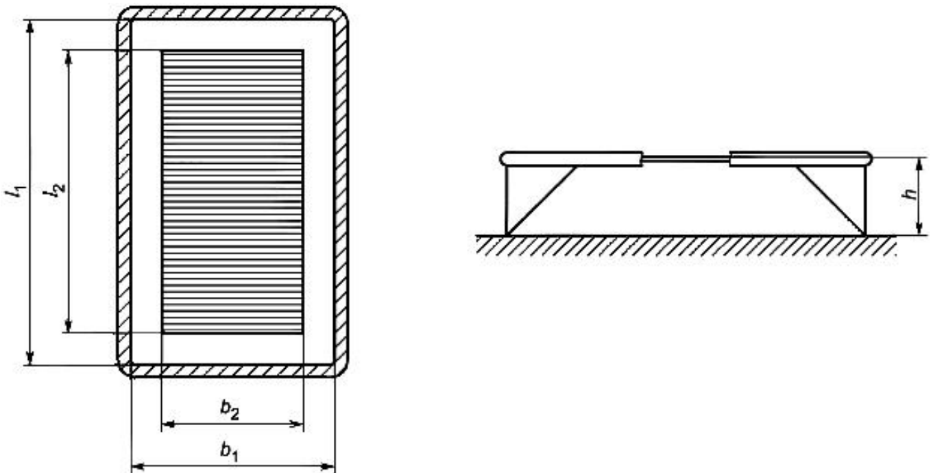
Рисунок 1 - Размеры батутов класса 1
