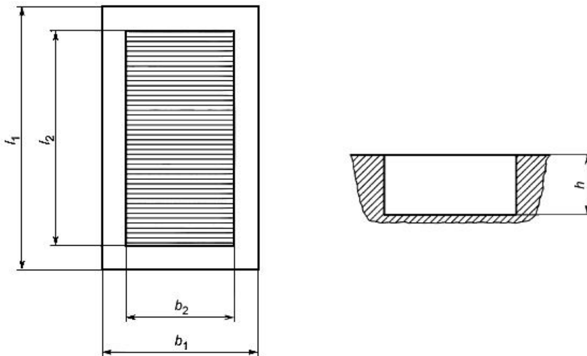
Рисунок 5 - Размеры батуты класса 5
