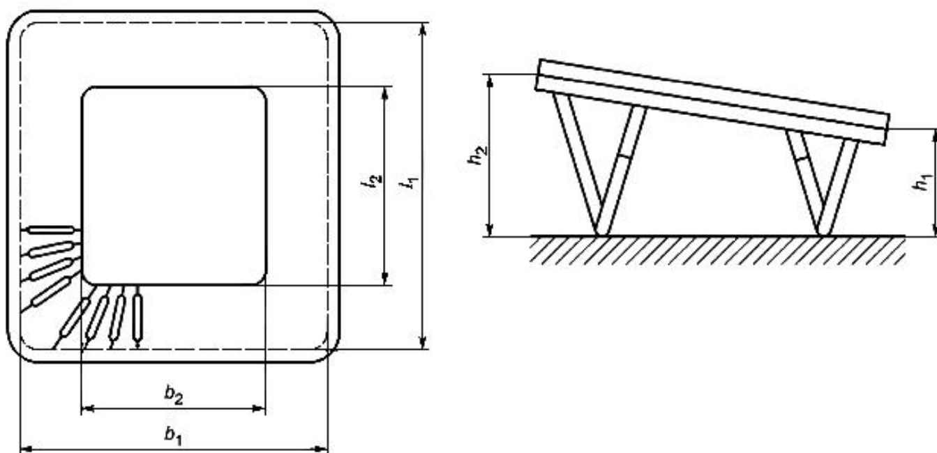
Рисунок 2 - Размеры батутов класса 2
